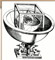
Mysterium Cosmographicum (1600)
